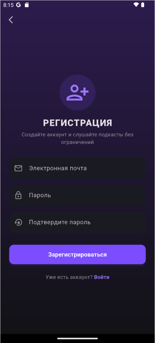
Рисунок 5.2 – экран регистрации
